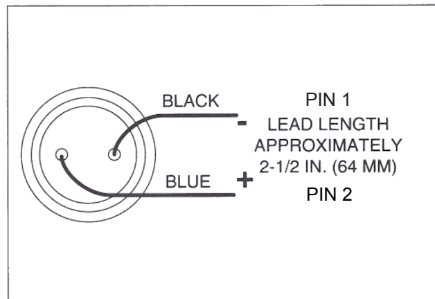
Wiring Diagrams
